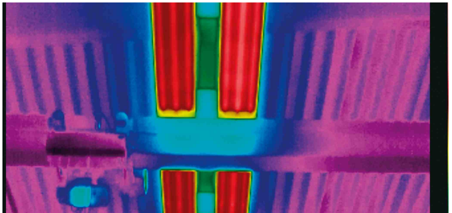
Die Thermografie-Aufnahme zeigt die thermische Entkoppelung der Strahlfläche von den LED-Leuchten.
