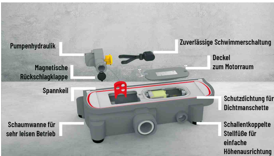
Der Aufbau der Plancofix Connect.
